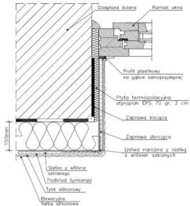
DETAL OCIEPLENIA OŚCIEŻA OKIENNEGO I DRZWIOWEGO
