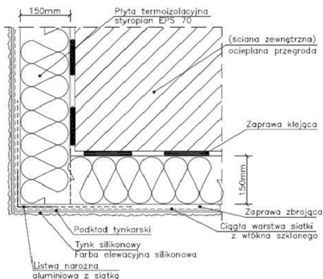
DETAL OCIEPLENIA NAROŻA WYPUKŁEGO
