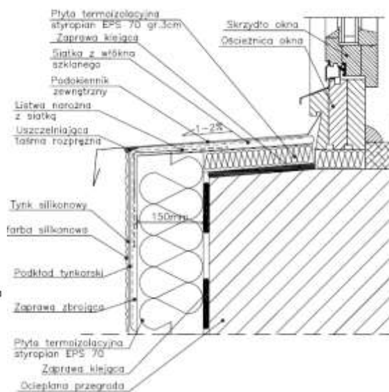
DETAL ZAMOCOWANIA PODOKIENNIKA
